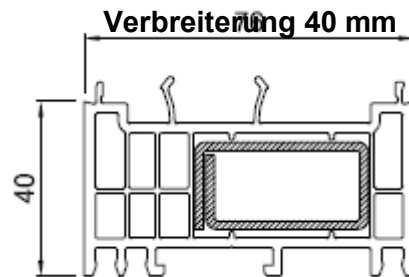
40 mm Nr. 416164
