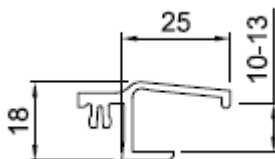
Kastenanschluss Nr. 406053
