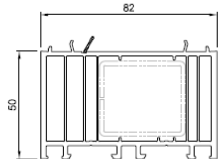
50 mm Nr. NP8500 Verstärkung Nr. VS3030
