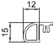
Abrollleiste Nr. 406051
