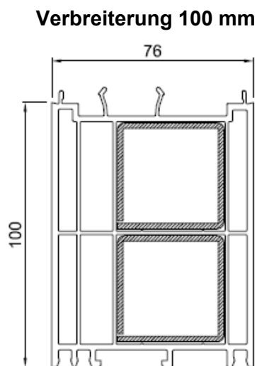
100 mm Nr. 416176
