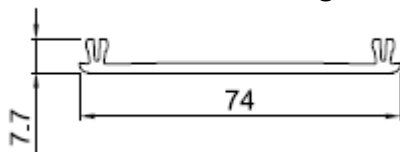
Abdeckung Nr. 416180
