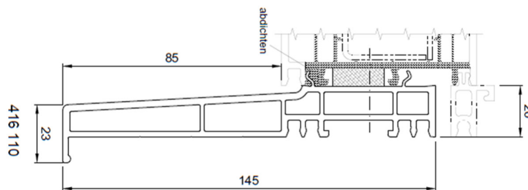
FBA Nr. 416110
