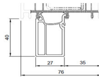
FBA Nr. 416141
