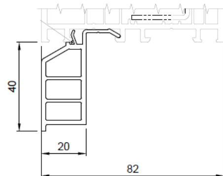
Anschlussituation 40 mm
