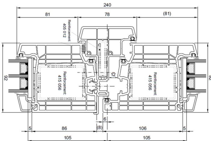
Flügel Nr. 171 040 – Stulp Nr. 176 020
