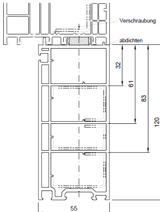
Anschlusssituation 120 mm
