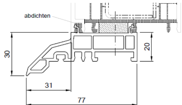
FBA Nr. 416126
