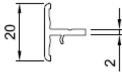
Kopplungs Nr. NP0190
