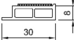
Abdeckleiste weiss Nr. 416337 Abdeckleiste foliert Nr. 640736
