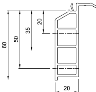
FBA Nr. NP0380
