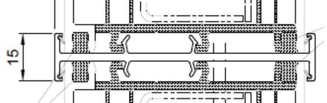
Anschlussituation H-Kopplungsprofil
