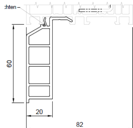
Anschlussituation 60 mm
