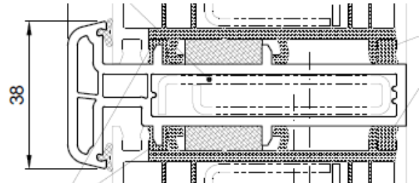
Anschlussituation Statikkopplung 15 mm
