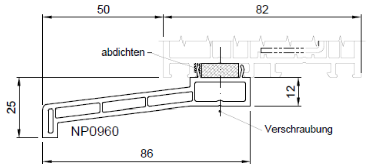
Anschlusssituation 86 x 25 mm
