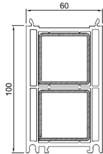
100 mm Nr. 406176
