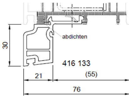
FBA Nr. 416133
