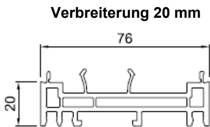
20 mm Nr. 416160
