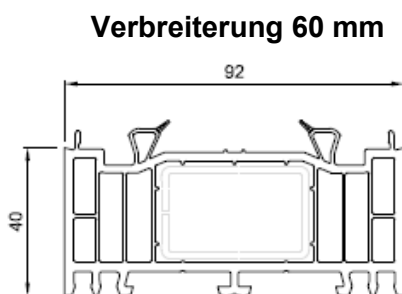
60 mm Nr. 476164
