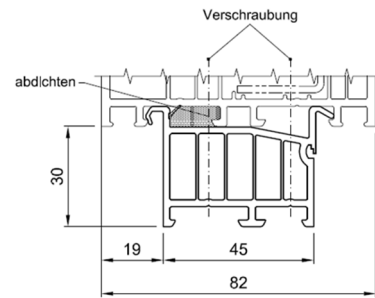
Anschlusssituation FBA 30 mm
