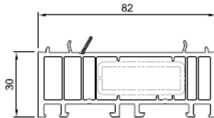
30 mm Nr. NP8300 Verstärkung Nr. VS4020
