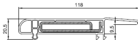
Anschlussprofil Nr. 476055
