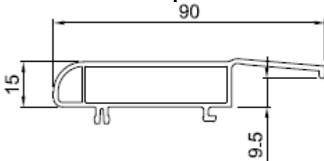
Anschlussprofil Nr. 416055
