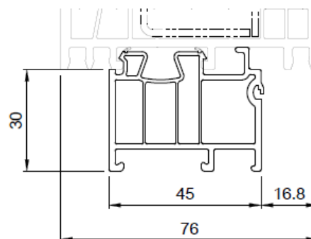
FBA Nr. 416106
