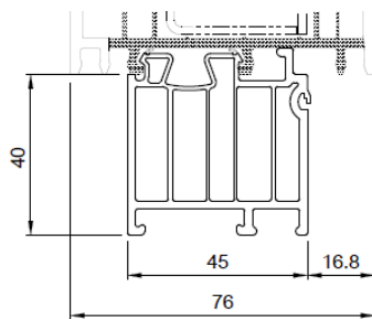
FBA Nr. 416100
