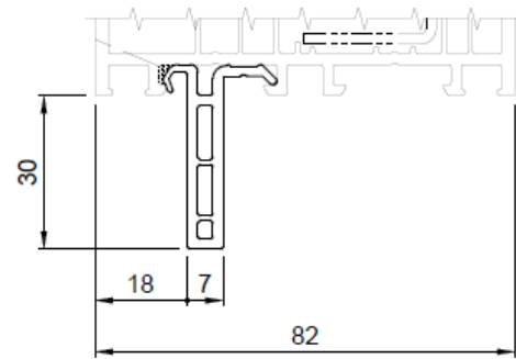
Anschlussituation 30 mm
