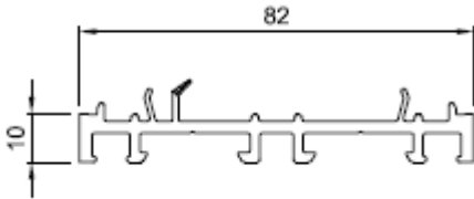
10 mm Nr. NP8200
