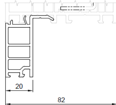
Anschlussituation 40 mm
