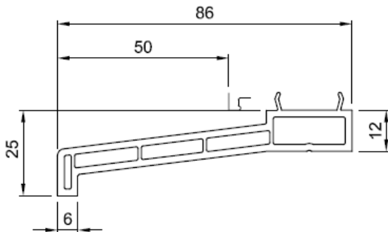
FBA Nr. NP0960
