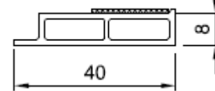
Abdeckleiste weiss Nr. ZF2080 Abdeckleiste foliert Nr. 640746
