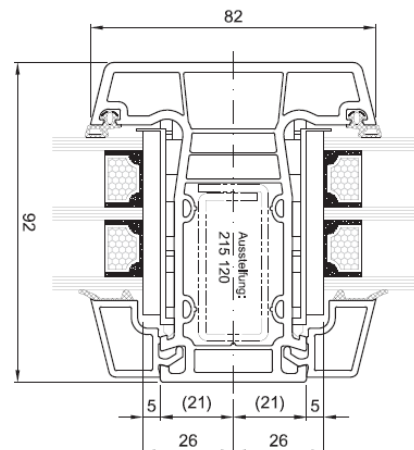
Sprosse Nr. 172425
