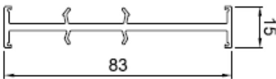
Kopplungs Nr. 416260
