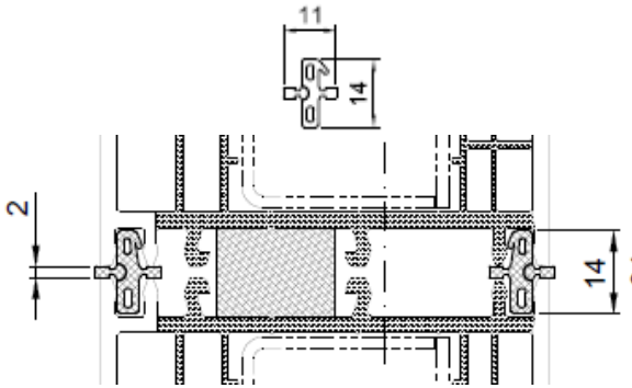
Kopplungs Nr. 414915
