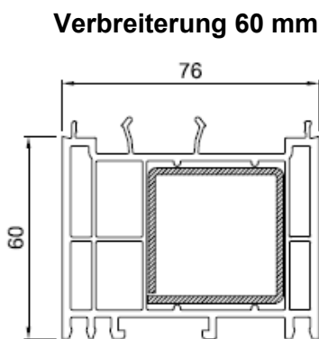
60 mm Nr. 416170
