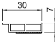
Kammerprofil Nr. 640736
