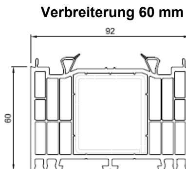
60 mm Nr. 476170
