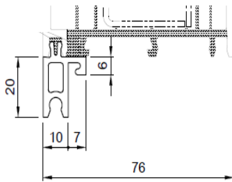
FBA Nr. 406105
