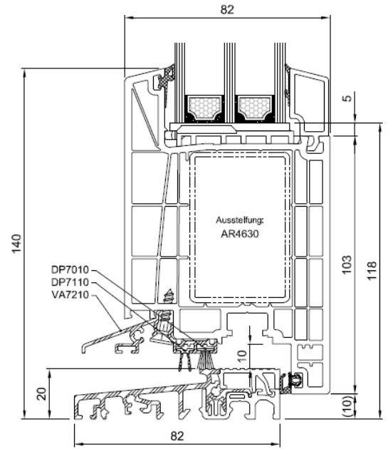
Flügel Nr. HP 8550
