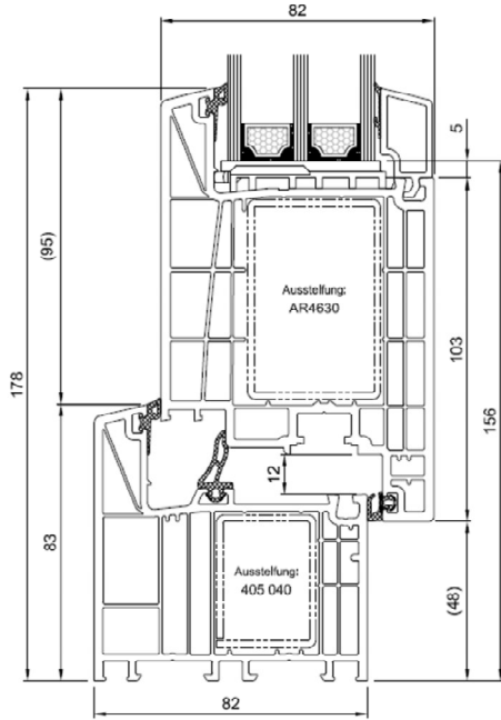
Blendrahmen Nr. HO 9030 – Flügel Nr. HP 8550
