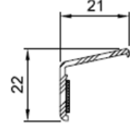
Trittschutz Nr. 476620
