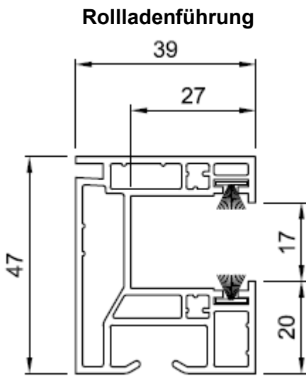
Rollladenführung Nr. RF0530
