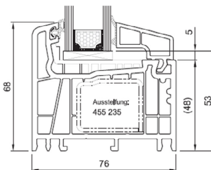
Festverglasung Nr. 250 221
