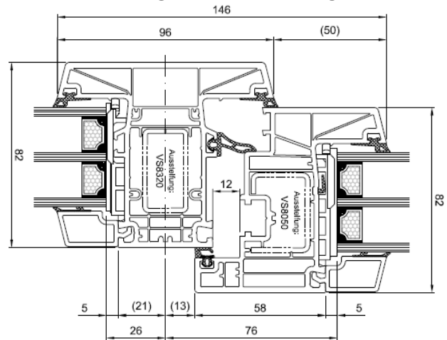
Festverglasung HO 9320 – Flügel HO 8520
