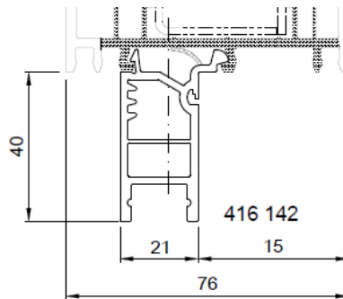
FBA Nr. 416142
