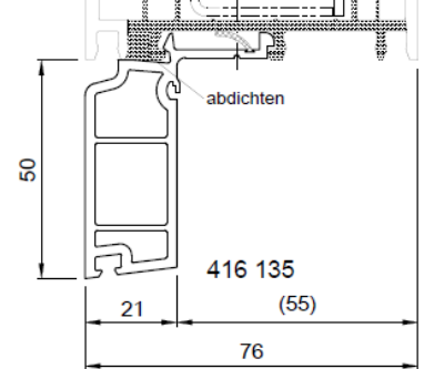
FBA Nr. 416135
