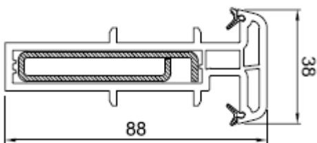
Kopplungs Nr. 416272
