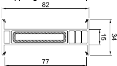
Kopplungs Nr. 416273
