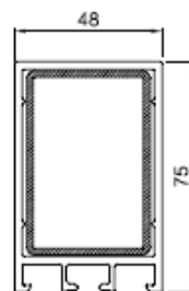
Lisene Nr. 416269 + 9023510
