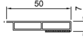
Kammerprofil Nr. 640756
