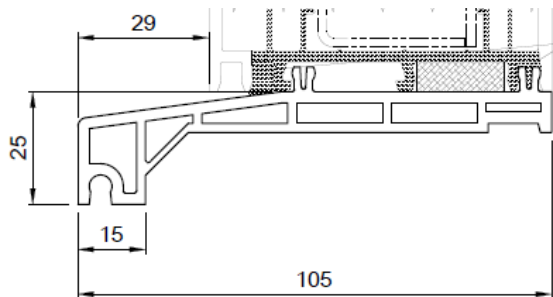
FBA Nr. 406115
