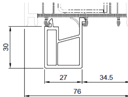
FBA Nr. 416131
