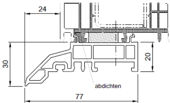
FBA Nr. 416126
