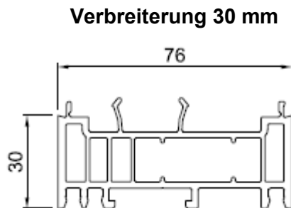
30 mm Nr. 416163
