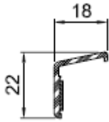
Trittschutz Nr. 216620
