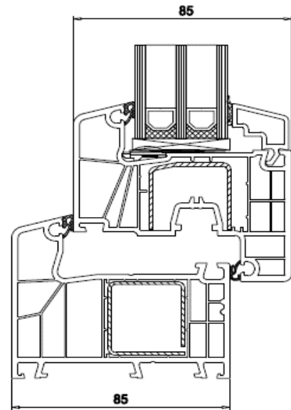
Zugrundeliegende Profil-Kombination für Uf
